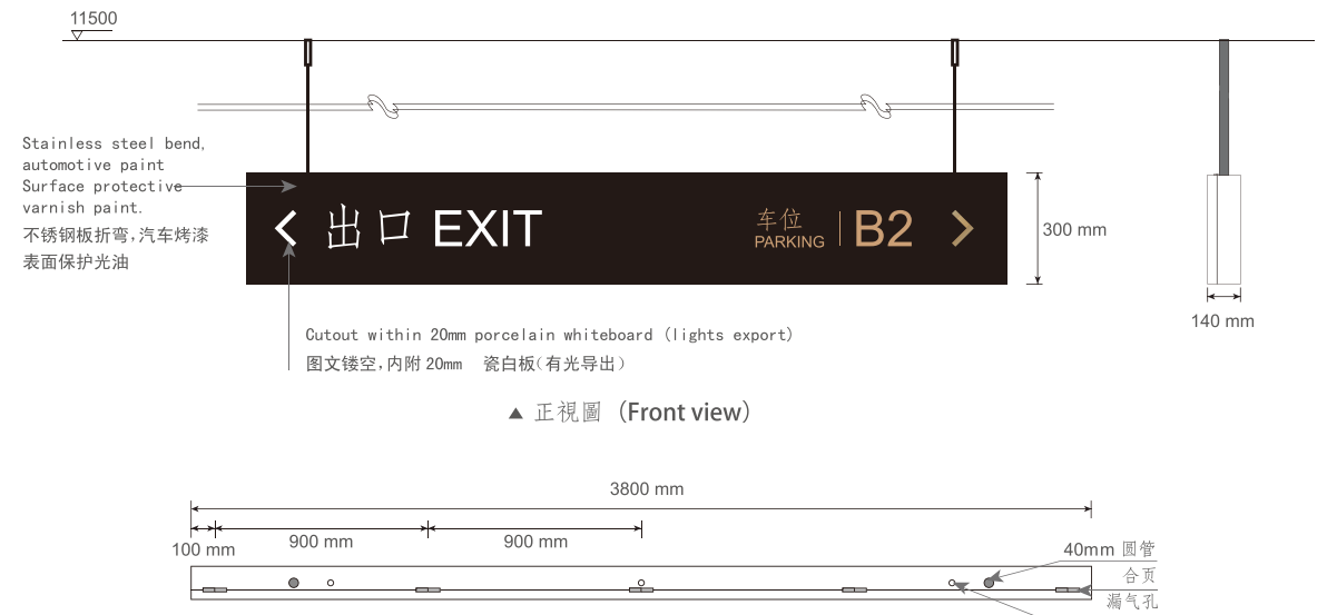
▲ 顶视图 (Top view)
