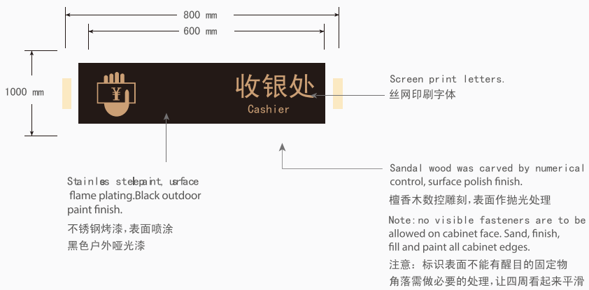
▲ 正视图 (Front view)
