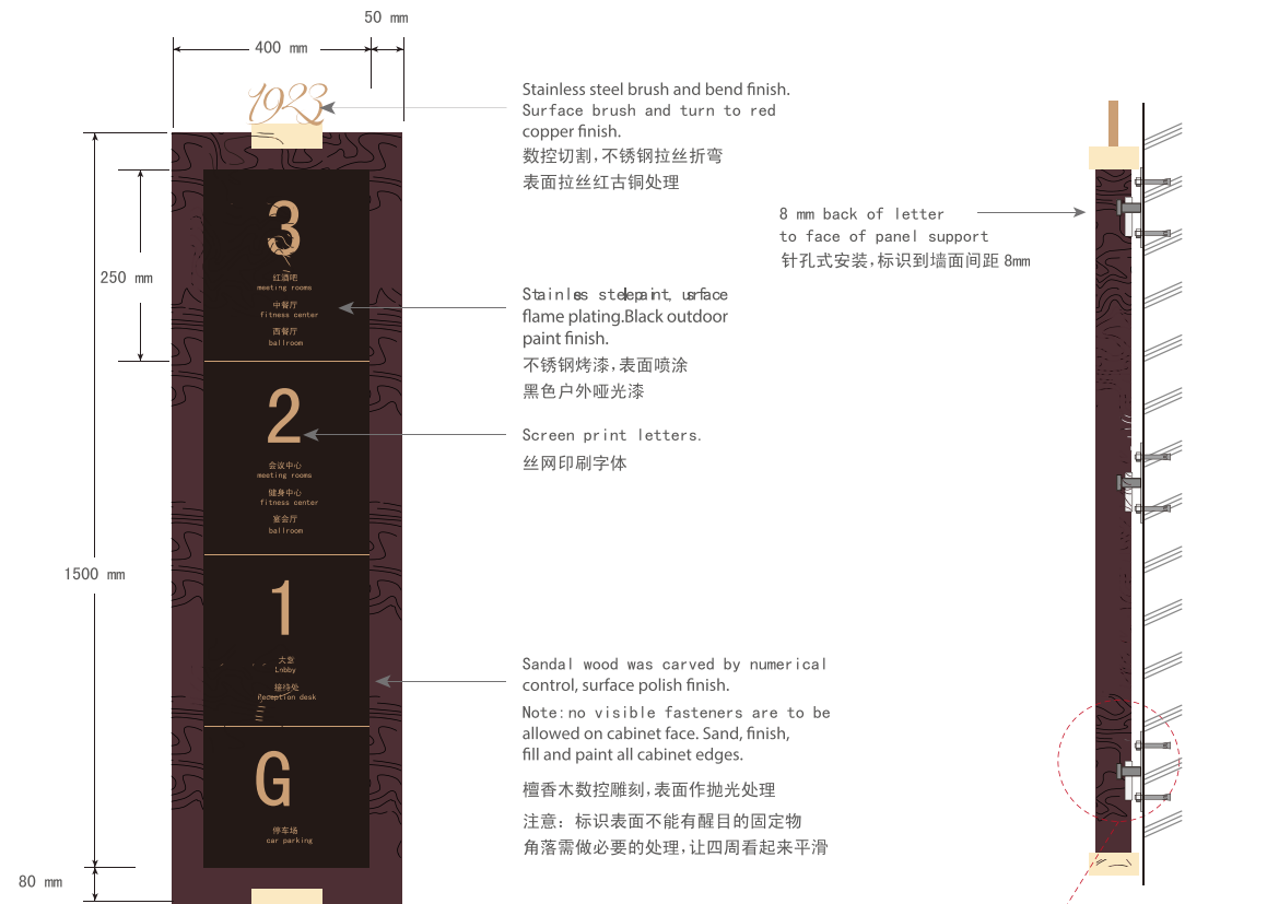
▲ 侧视图 (Side view)
