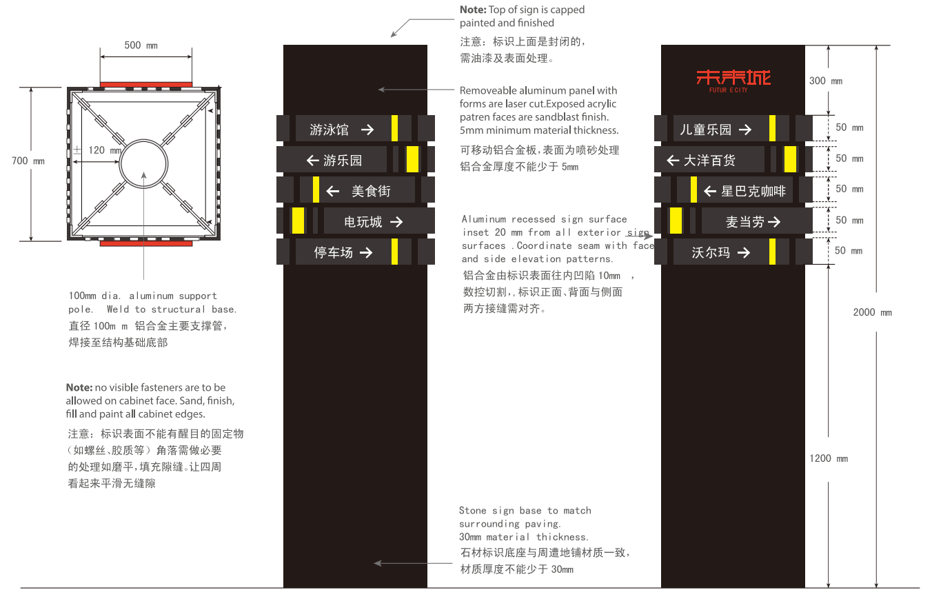
▲ 正视图 (Front view)
