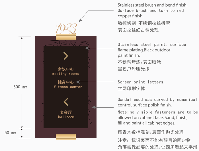
▲ 正视图 (Front view)
