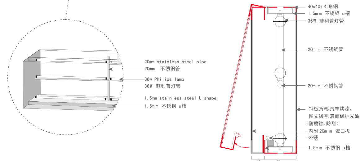
▲ 细节图 (Detail view)
