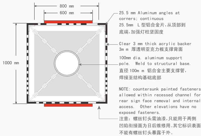
▲ 顶视图 (细节) (Top view)
