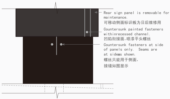
▲ 底座侧面图 (细节) (Base Side view)
