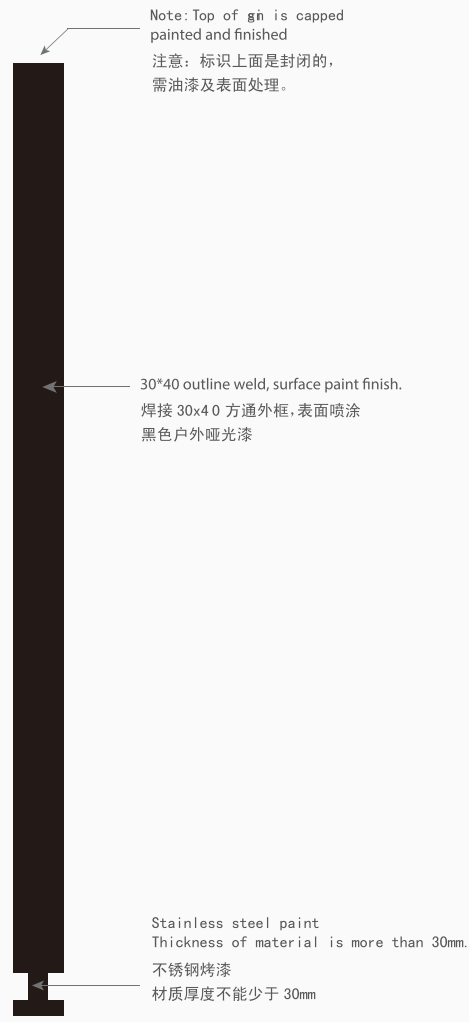
▲ 侧视图 (Side view)
