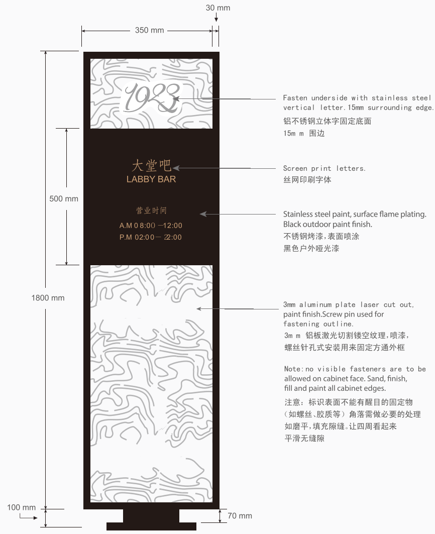
▲ 正视图 (Front view)
