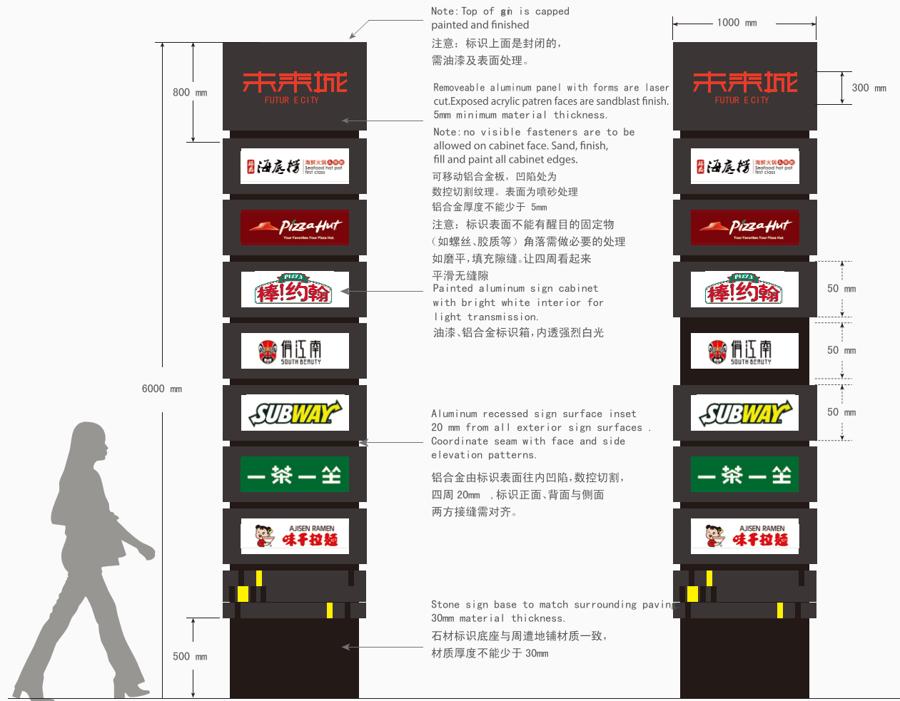
▲ 正视图 (Front view)
